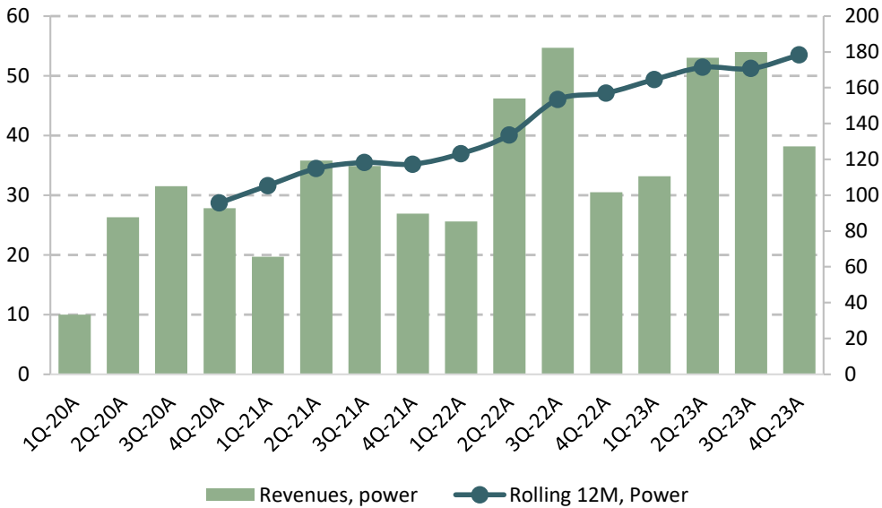
Figur 1: Försäljning, el, kvartalsvis och rullande 12M
