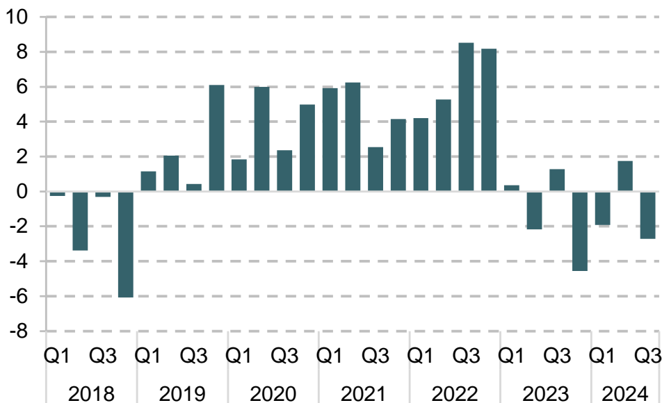
Figur 1: EBIT, kvartalsvis
